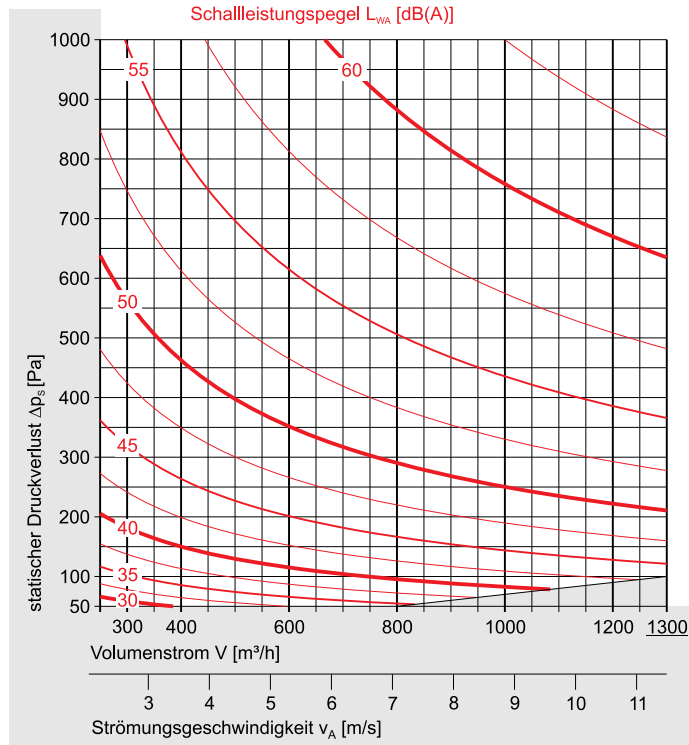
Größe DN 200
