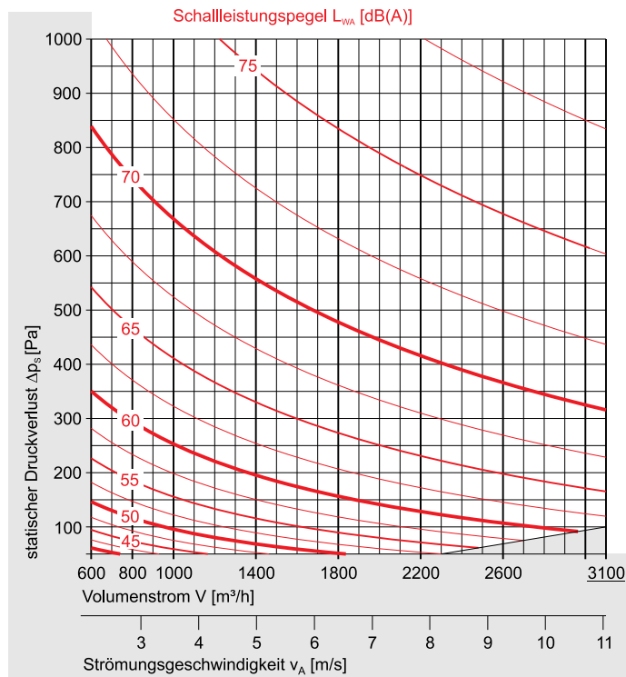
Größe DN 315
