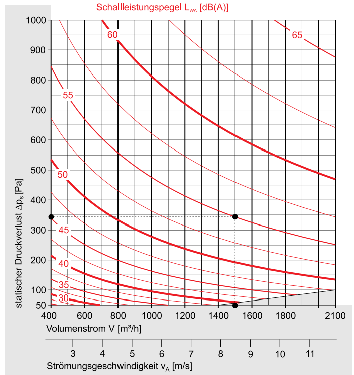
Größe DN 250
