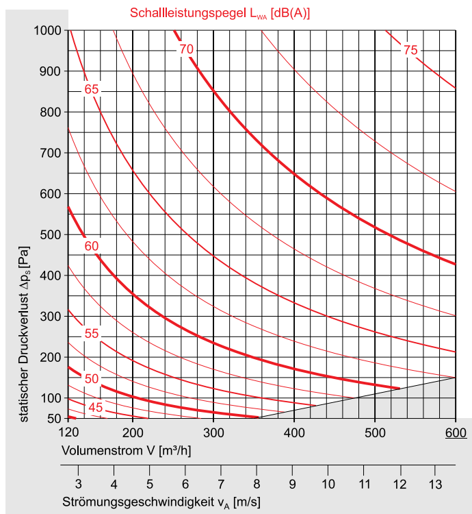
Größe DN 125
