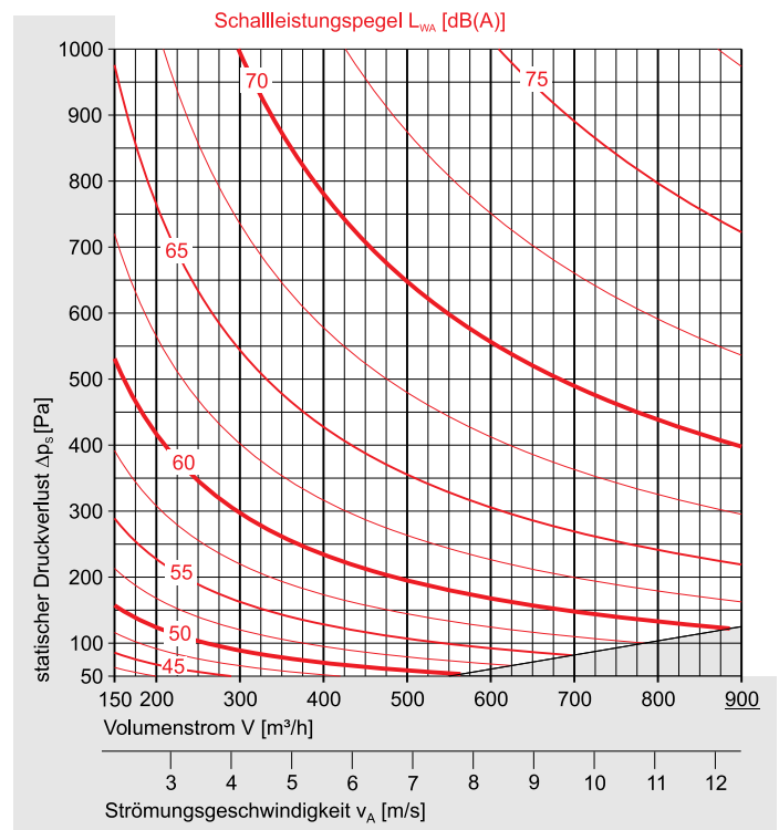
Größe DN 160
